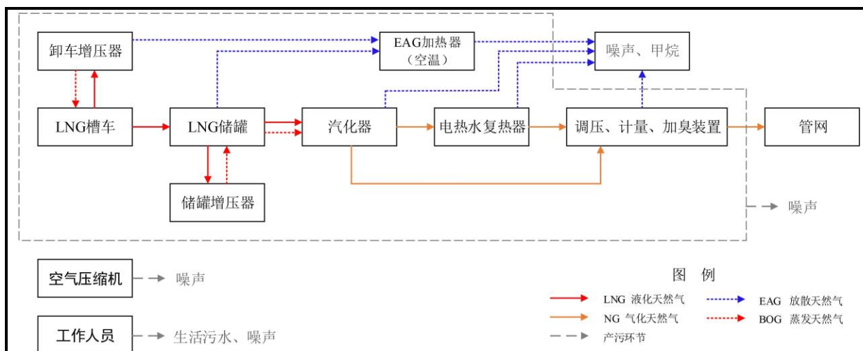
图4 运营期工艺流程及污染物排放
