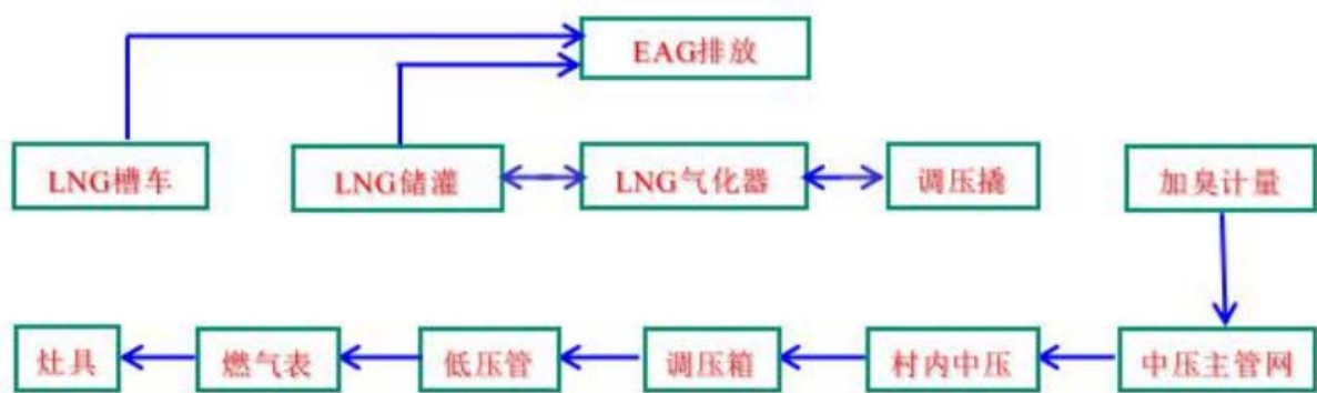
图 2 拟建项目工艺流程图
